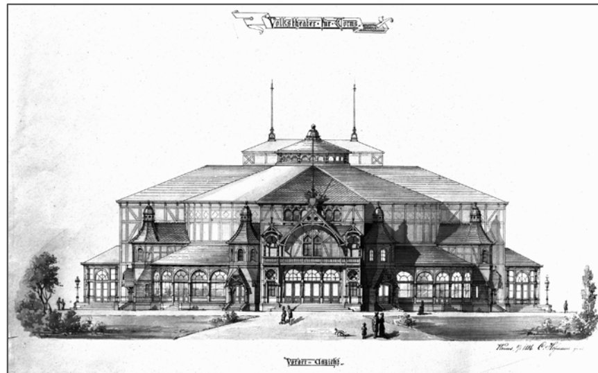
Entwurf "Volkstheater Worms" von C. Hoffmann, Januar 1886 Vorderansicht
